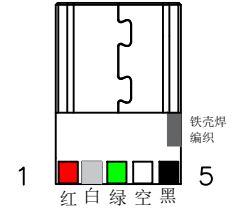
Micro usb母头焊接面
