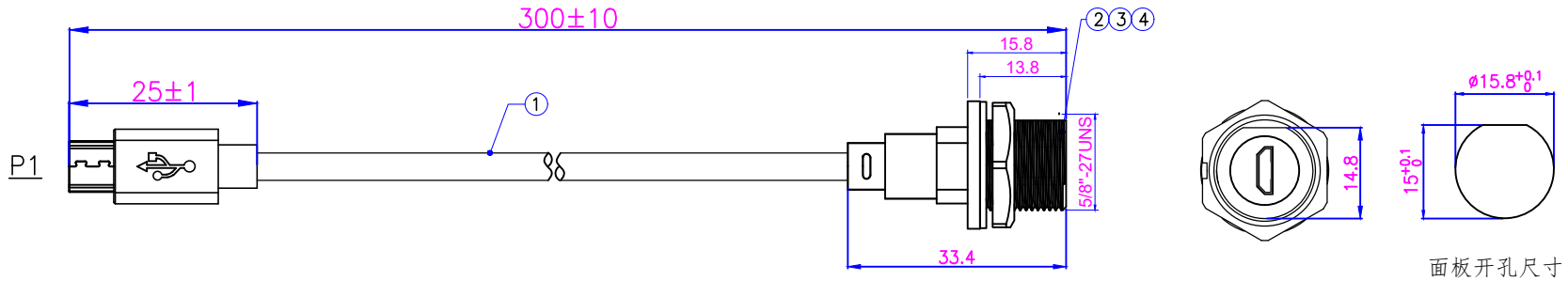
面板开孔尺寸
