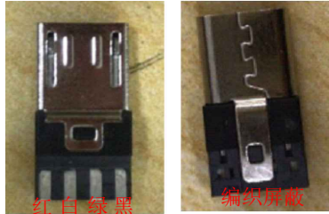
公头线束焊接实物图
