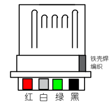
Micro usb公头焊接面
