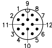
12Pin
