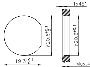
面板开孔尺寸
