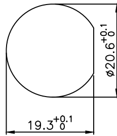
面板开孔尺寸
