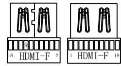
母头焊接面
