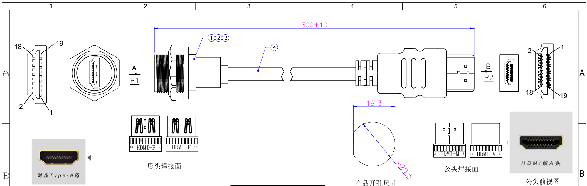
母头前视图
