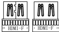
母头焊接面
