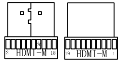
公头焊接面
