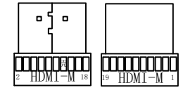
公头焊接面
