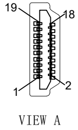
公头焊接面
