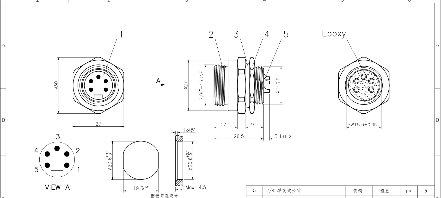
面板开孔尺寸
