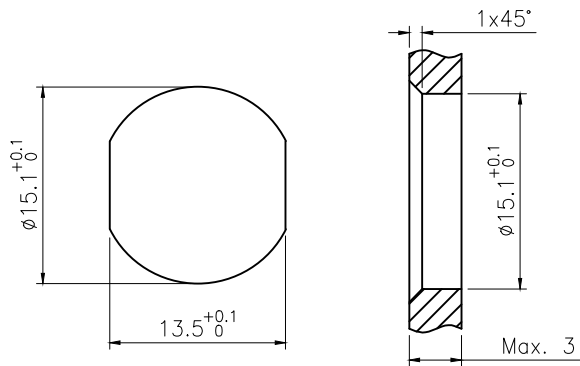
面板开孔尺寸
